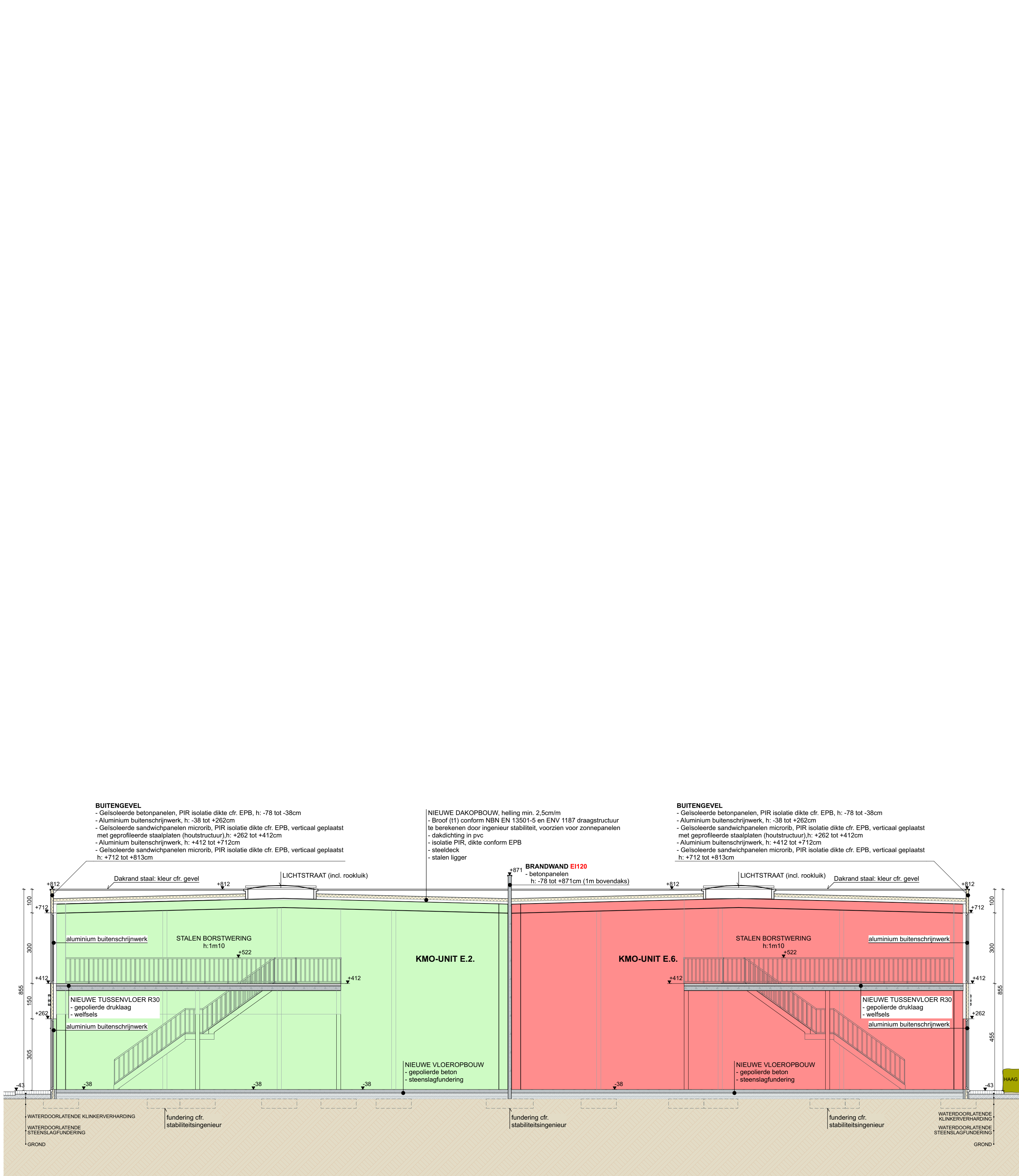
SB SNEDE B - NIEUWE TOESTAND BRAND 1:100
